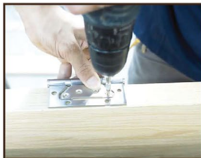
Bước 5: Bắn 3 bản lề vào cánh cửa theo đúng khoảng cách quy định
