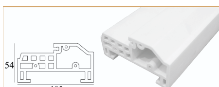
Phôi đồ cửa Pima PAK-105 Pima Door Profile PAK-105 1950-2300 x 105 x 54
