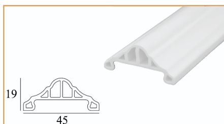
Nạp viền trang trí thất lũng PWA 45-20 Pima Decorative Trim PWA 45-20 3000 x 45 x 19
