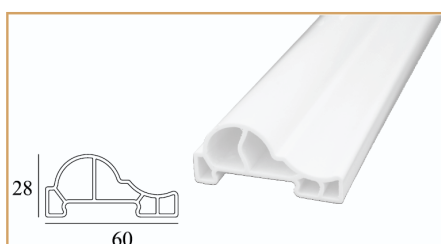
Nạp viền trang trí PWA 60-28 Pima Decorative Trim PWA 60-28 3000 x 60 x 28
