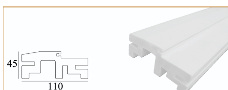
Phôi đồ cửa Pima PATB-110 Pima Door Profile PATB-110 1950-2300 x 110 x 45
