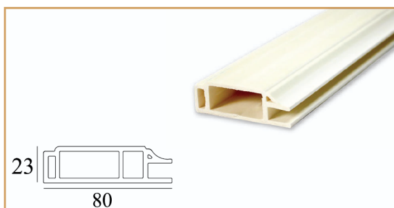
Thanh đồ cánh tủ PMK 8023 Cabinet Door Profile PMK 8023 3000 x 80 x 23
