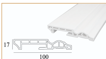
Nạp trang trí chân tường PWA 100-17 Pima Decorative Footing Trim PWA 100-17 3000 x 100 x 17
