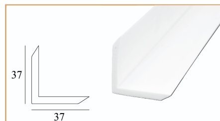
Nạp viền trang trí PVN 37-37 Pima Decorative Trim (V EXTERNAL ANGLE) PVN 37-37 3000 x 37 x 37
