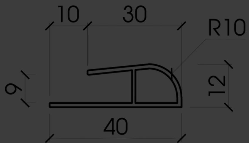
NẸP KẾT THÚC ECK 30 - 40
