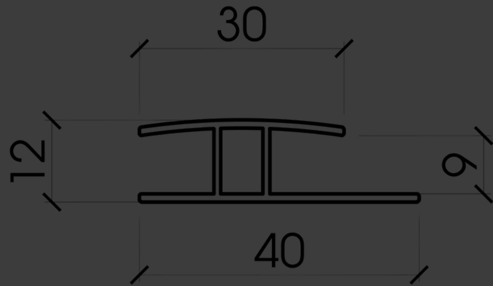
NẸP NỐI CHỮ H, ECN 30 - 40
